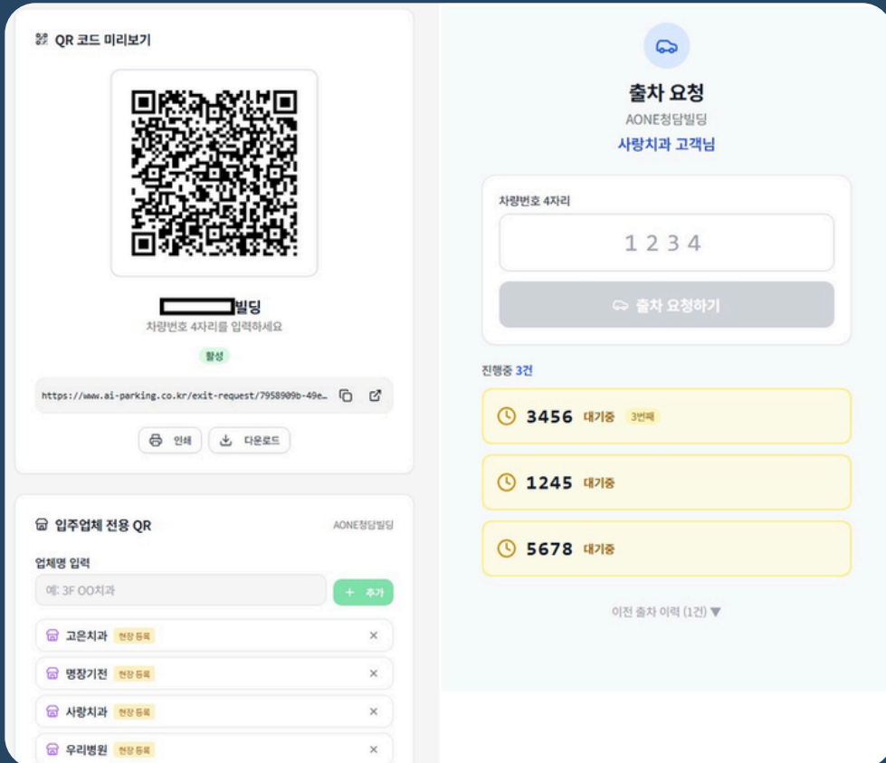
QR 출차 요청 — 입주업체별 관리, 실시간 상태 추적, QR 코드 인쇄
