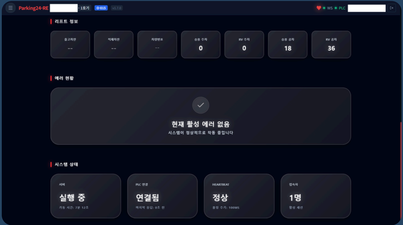
실시간 대시보드 — PLC 상태, 오늘의 통계, 활성 에러, 접속자 정보
